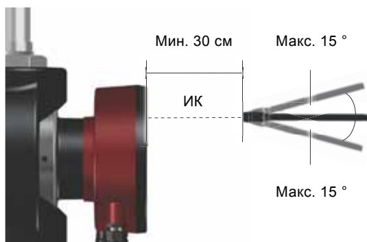
Рис. 31 ИК-соединение между Grundfos GO и MAGNA1
